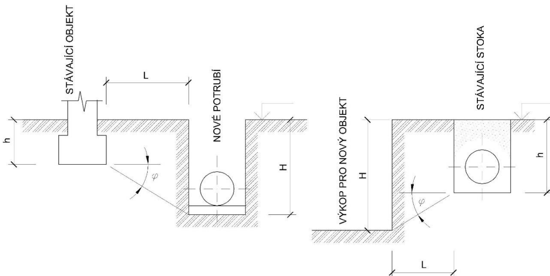
Obrázek 4 – Bezpečná vzdálenost mezi dnem konstrukce stoky a obrysem základu budovy
